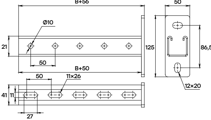
STRUT-консоль 41x41
