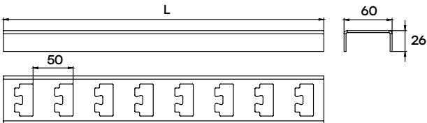
Стойка кабельная
