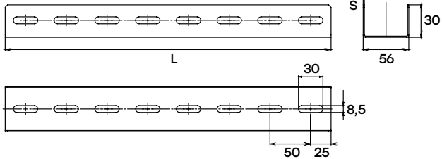
Профиль П-образный
