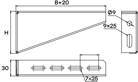
Кронштейн настенный
