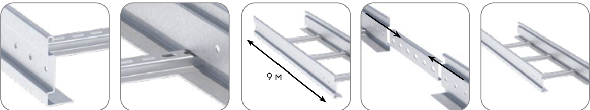
Усиленный профиль лонжерона Увеличенная толщина Максимальная длина – 9 м Усиленное соединение при помощи пластин Удобное обслуживание кабельной трассы
