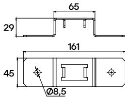
Скоба кабельная K1157
