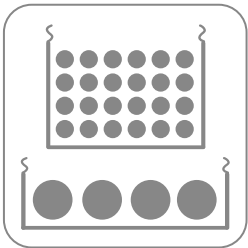
Сигнальный кабель рекомендуем укладывать в узкий лоток с высокой стенкой, силовой кабель - в широкий лоток с низкой стенкой
