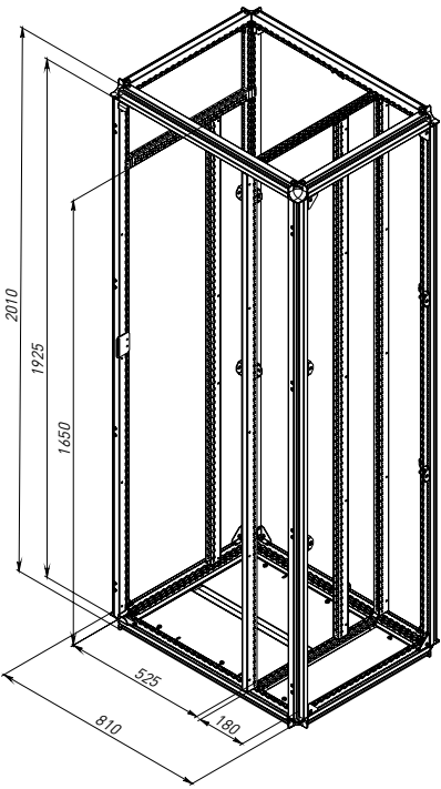
Глубина 600/800 мм (с дополнительными профилями)
