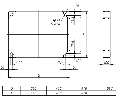
Крепление к полу
