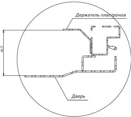
Полезное пространство за дверью
