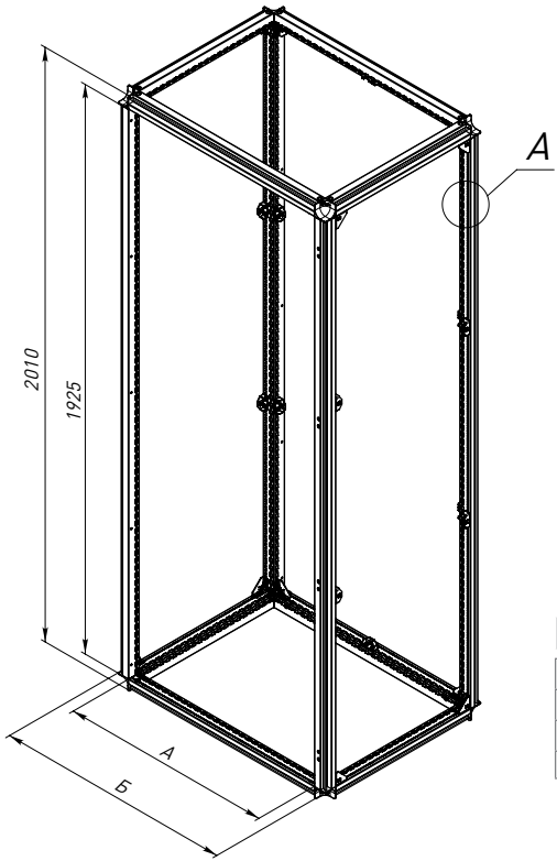
Глубина 600/800 мм (с дополнительными профилями)
