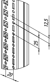
A (1:2) (перфорация профиля)
