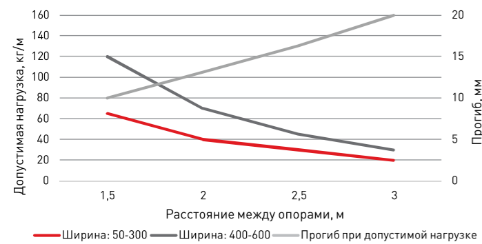
Графики нагрузки
