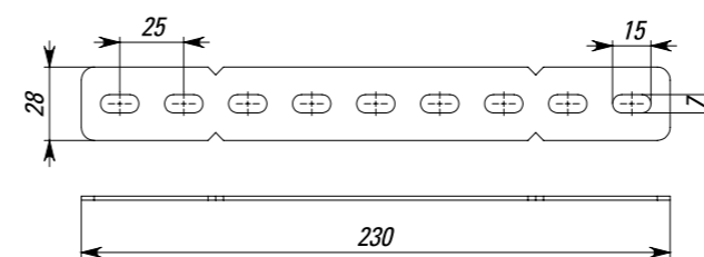
Перфорированный соединитель EKF
