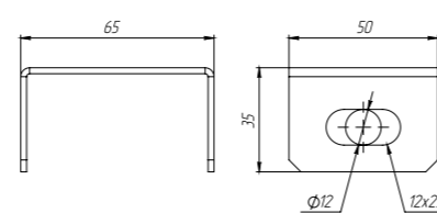
Держатель потолочный
