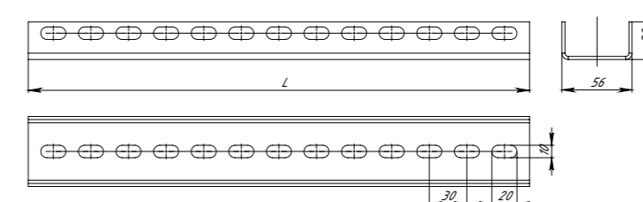
Профиль П-образный
