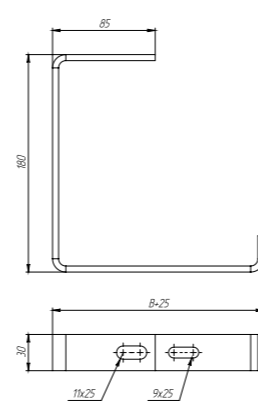
Подвес С-образный
