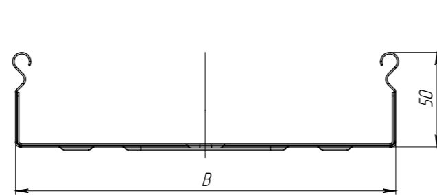
Габаритные размеры
