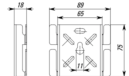
Плата монтажная универсальная EKF
