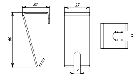
Фиксатор вертикальный EKF
