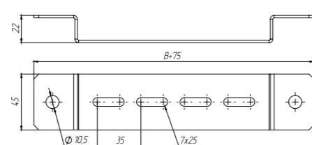
Скоба подвеса нижняя (стойка настенная)
