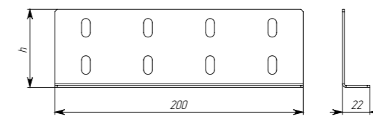
Пластина соединительная усиленная для лестничного лотка
