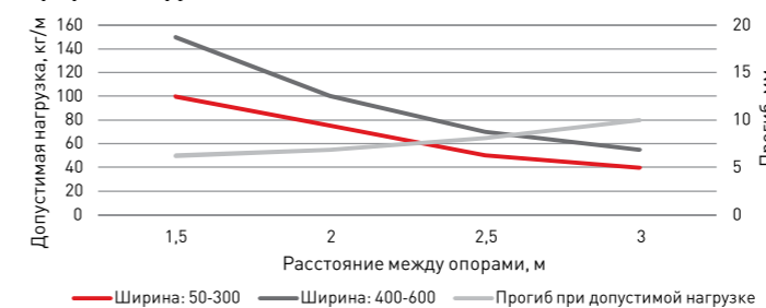
Графики нагрузки
