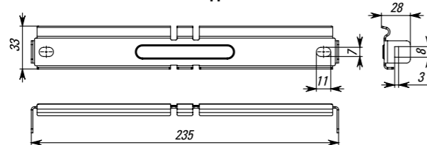
Безвинтовой соединитель EKF
