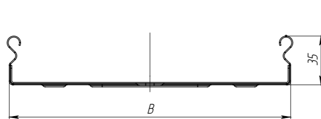
Габаритные размеры
