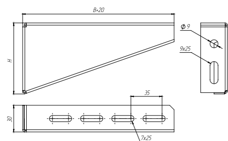
Кронштейн настенный
