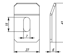
Прижим лестничного лотка EKF
