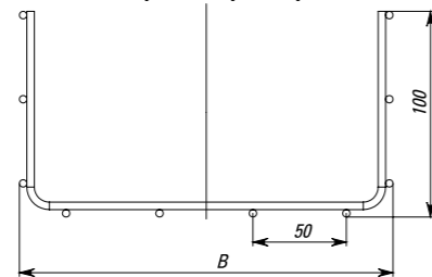
Габаритные размеры
