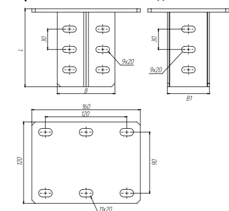
Кронштейн потолочный двойной
