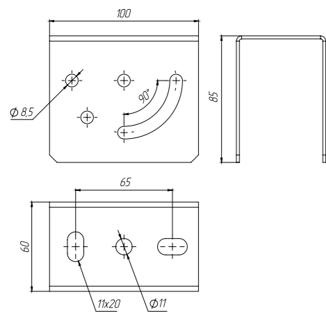
Скоба потолочная
