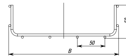
Габаритные размеры
