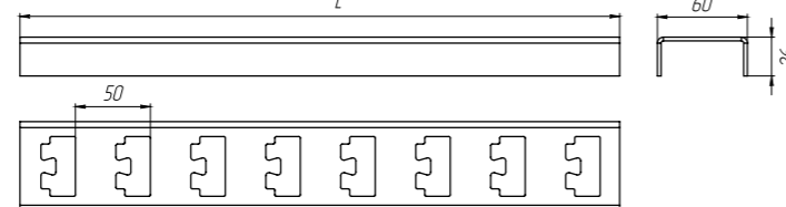
Скоба подвеса нижняя (стойка настенная)
