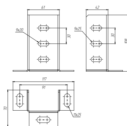
Кронштейн потолочный
