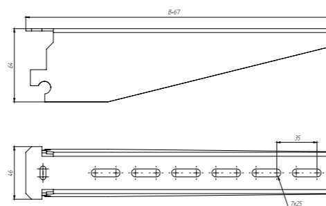
Полка кабельная
