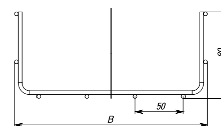
Габаритные размеры
