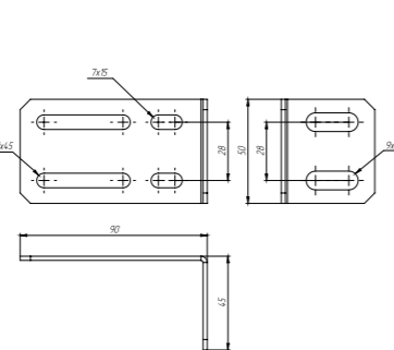
Кронштейн стеновой
