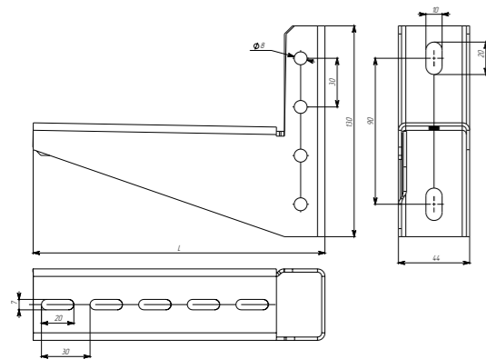
Кронштейн с опорой
