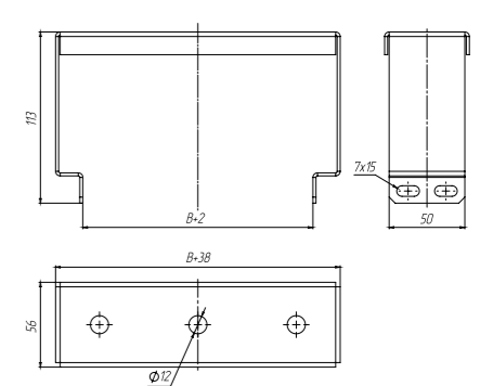
Скоба подвеса верхняя
