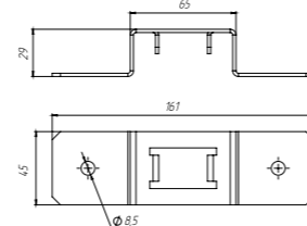
Скоба кабельная
